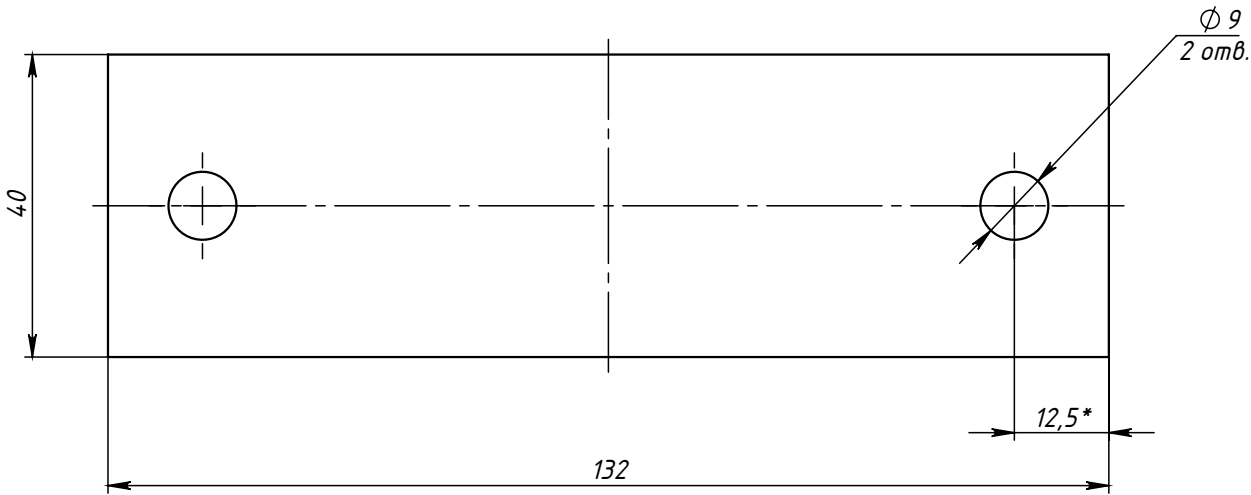
Поз.1 (Полухомут) развертка
