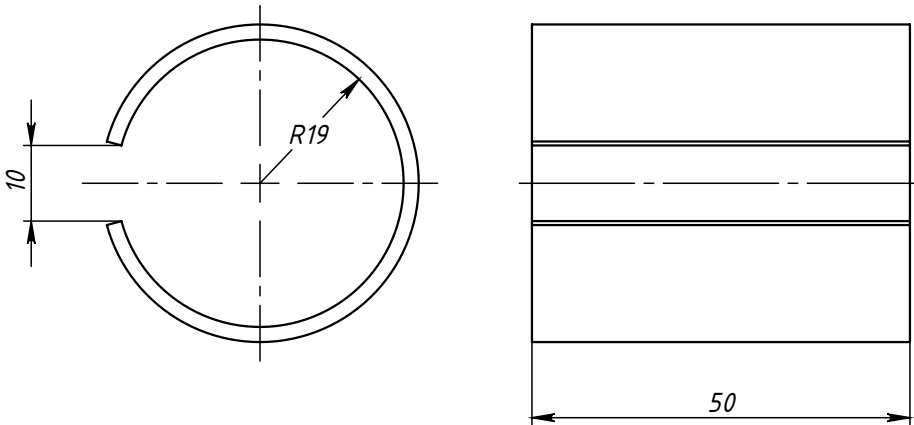
Поз.2 (Прокладка)
